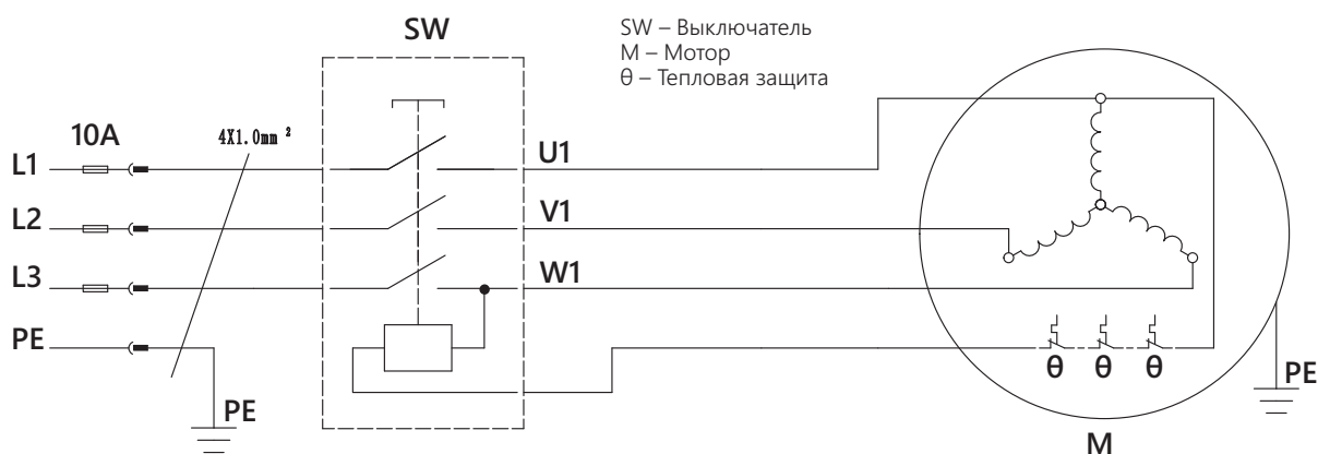
Рисунок 20. Модель BELMASH TS-250P/400 и BELMASH TS-250PE/400.
